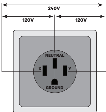
14-50R 240V/50A "RV" sortie.
