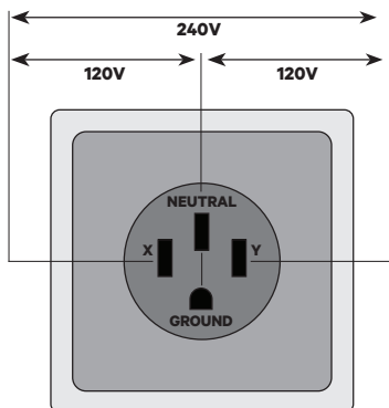
14-50R 240V/50A "RV" sortie.
