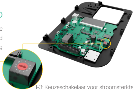
I-3: Keuzeschakelaar voor stroomsterkte
