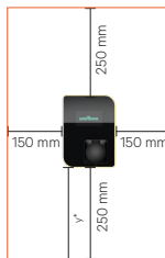
I-1: Monteringsyta
