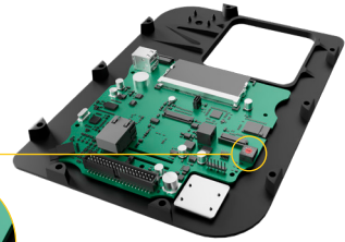
I-3: Stromwahlschalter
