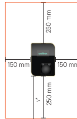
I-1: Montagefläche
