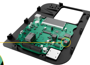
I-3: Selettore di corrente
