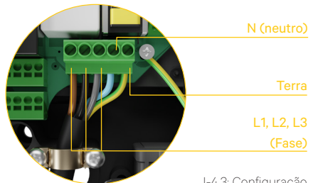
I-4.3: Configuração trifásica (3P)
