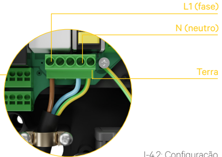
I-4.2: Configuração monofásica (1P)
