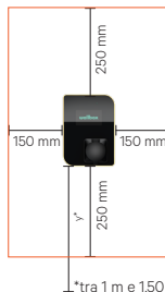
I-1: Area di montaggio
