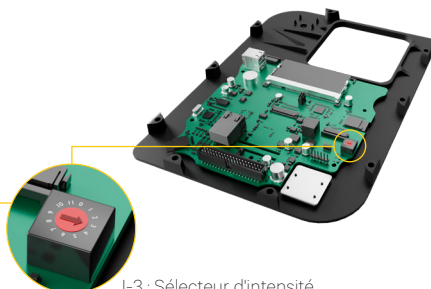
I-3 : Sélecteur d'intensité
