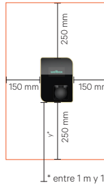
I-1: Zona de montaje
