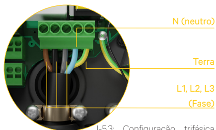
I-5.3: Configuração trifásica (3P)
