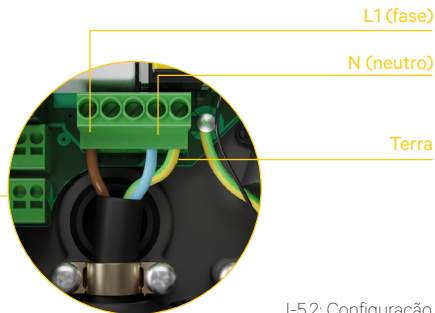
I-5.2: Configuração monofásica (1P)
