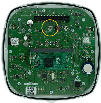
Fig. A.3.1 Impostazione dell'interruttore RS485 su "T"
