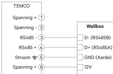
Fig. A2.2: Installatie bekabeling in Temco energiemeter
